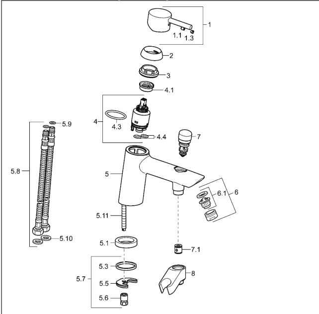
Výkres výrobku
