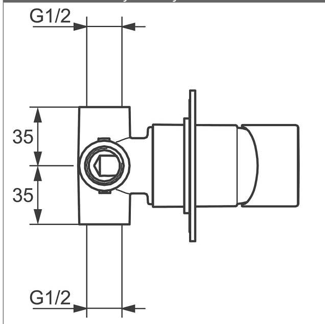
Výkres výrobku
